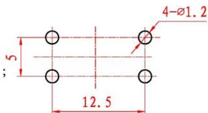
线路板安装孔图
